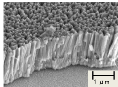
自己組織化した酸化チタンの柱状結晶 (直径 約200 nm, 長さ 1~2 μm)
