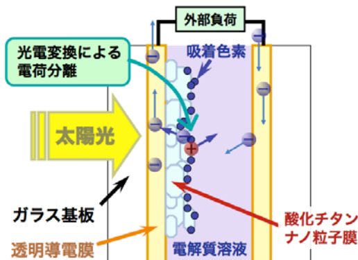
色素増感太陽電池の基本構造（模式図）
