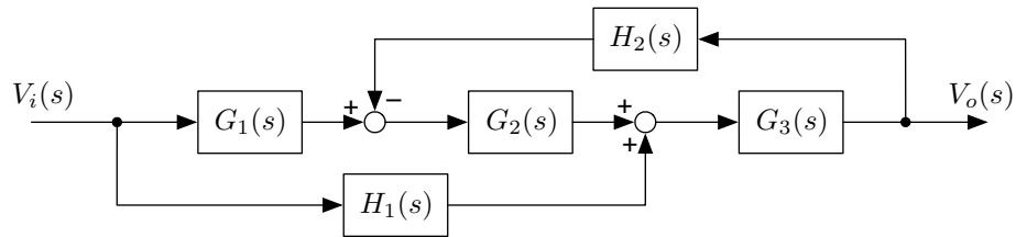
図：ブロック線図
